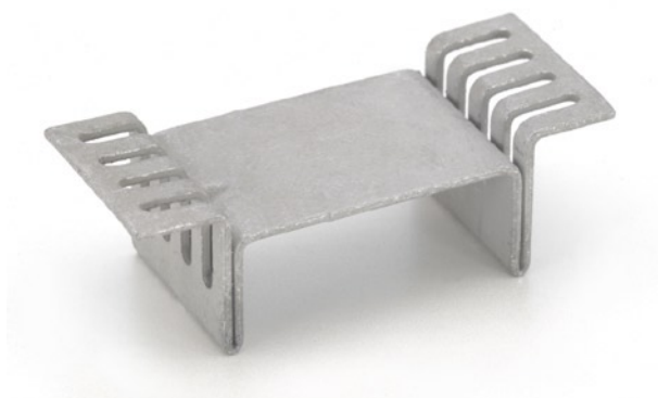
HS24 20°C/W
